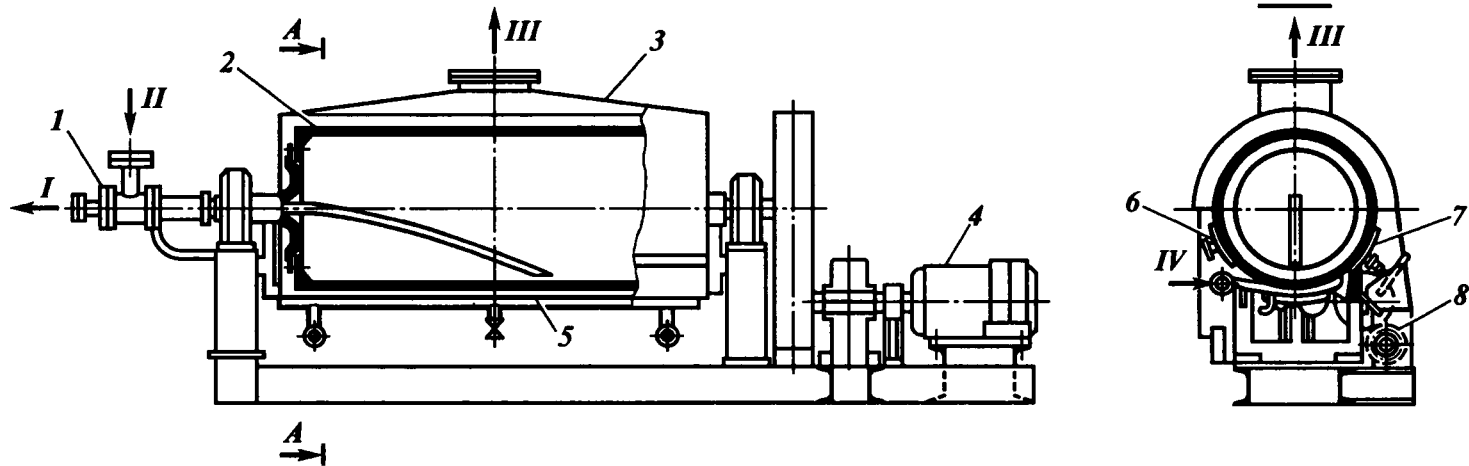
Рис. X-21. Одновальцовая сушилка:
